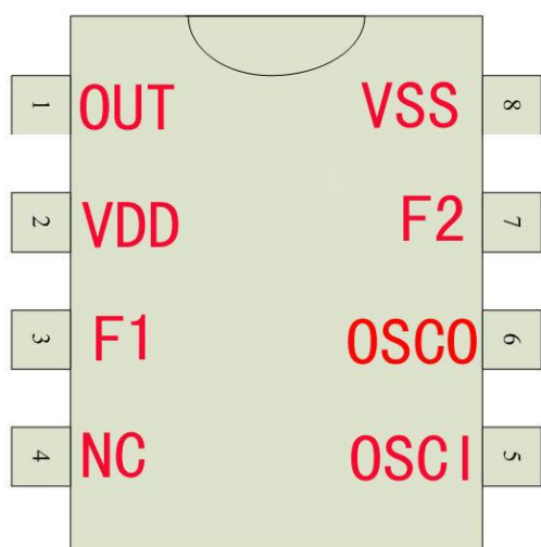
DIP8/SOP8 脚位
